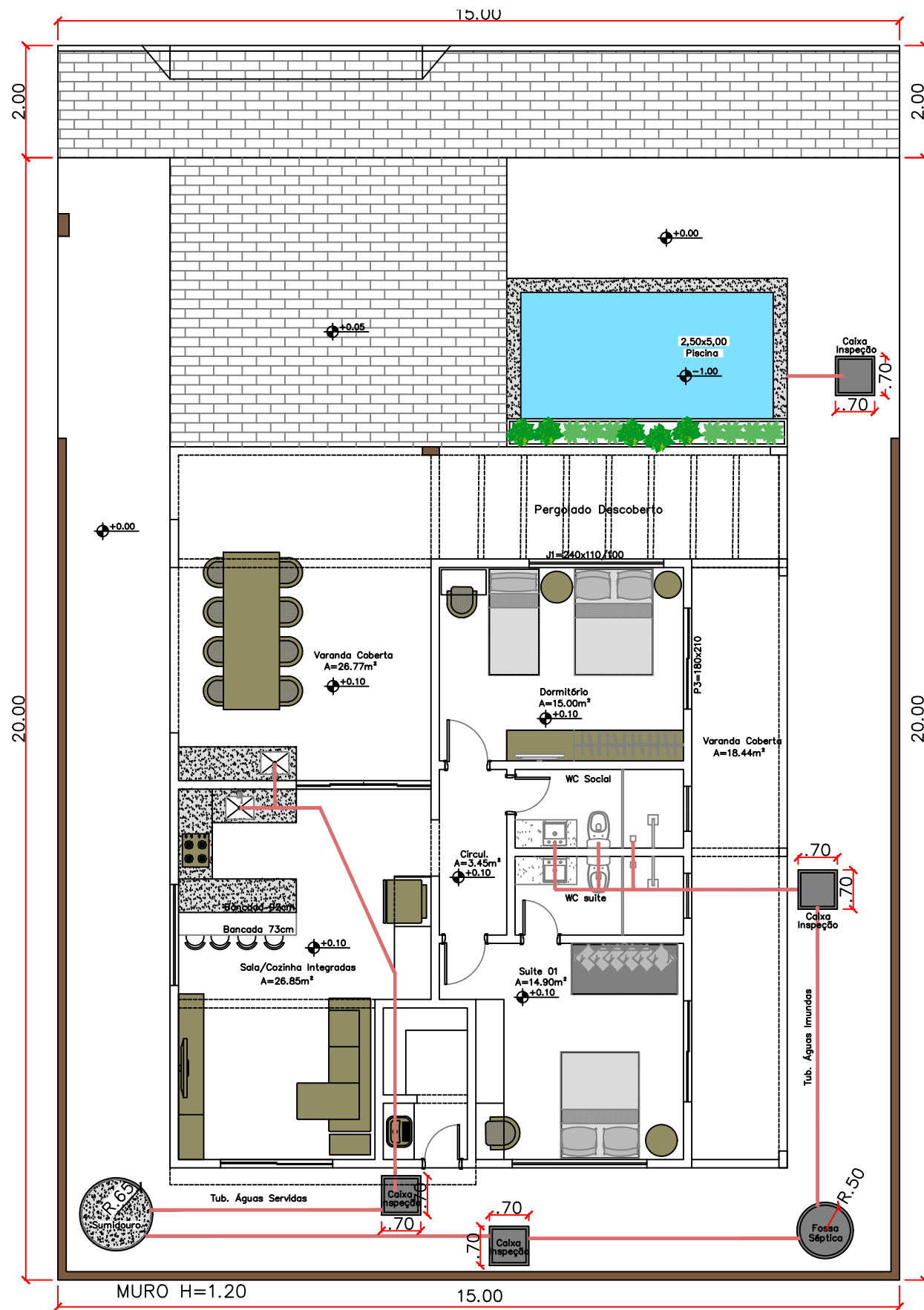
PLANTA BAIXA - FOSSA/SUMIDOURO Escala: _____ 1/100
