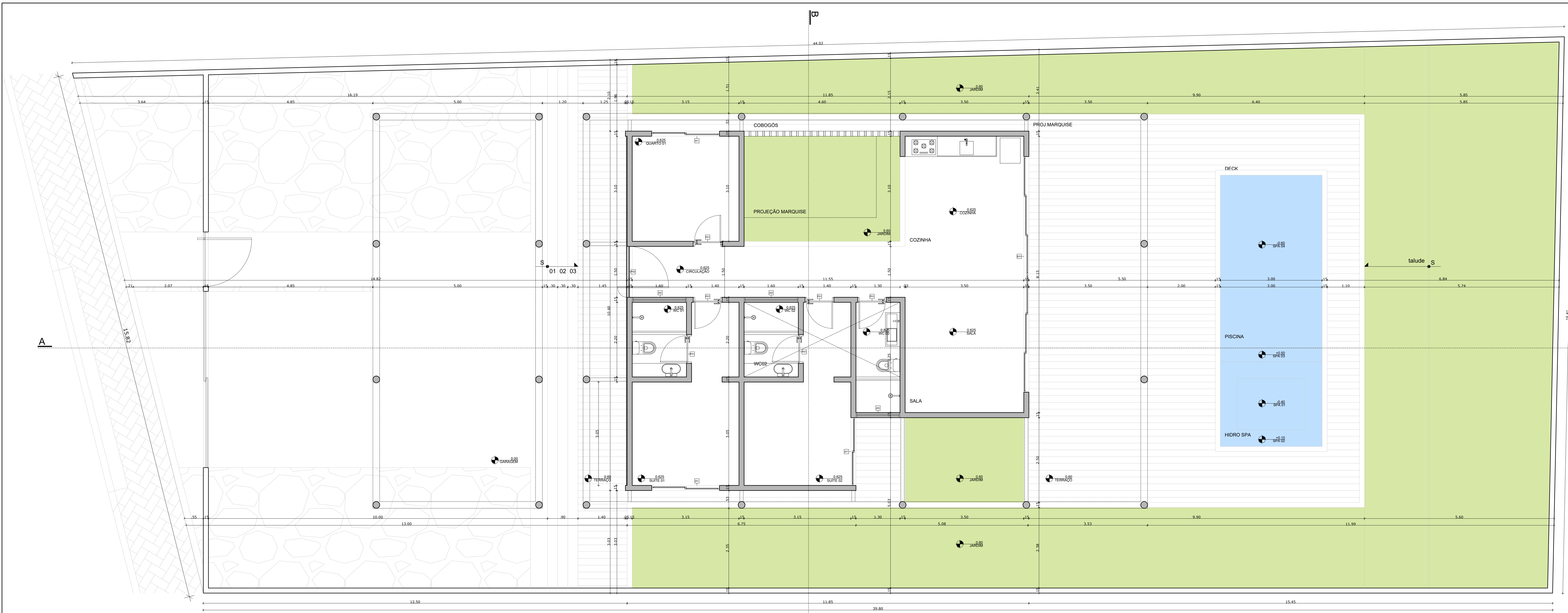
PLANTA BAIXA TERREO CHAGAS NETO ESCALA 1/50
