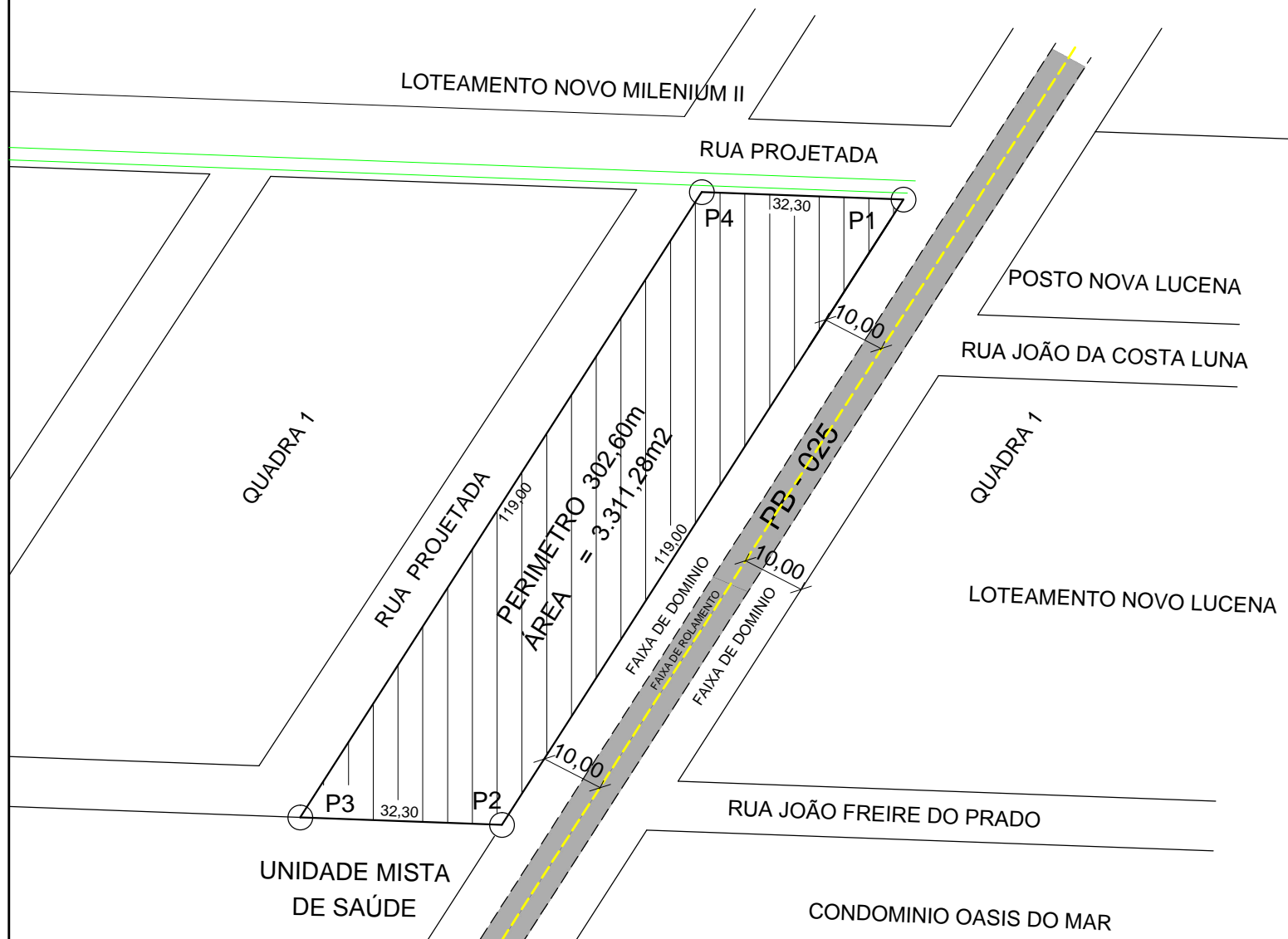
PLANTA DE SITUAÇÃO ATIAL ESCALA 1 / 1000
