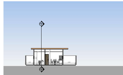
10 CORTE B ESCALA: 1/100
