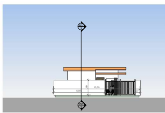
8 FACHADA SUL ESCALA: 1/100
