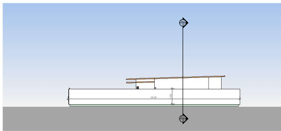
5 FACHADA LESTE ESCALA: 1/100
