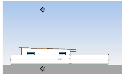
7 FACHADA OESTE ESCALA: 1/100
